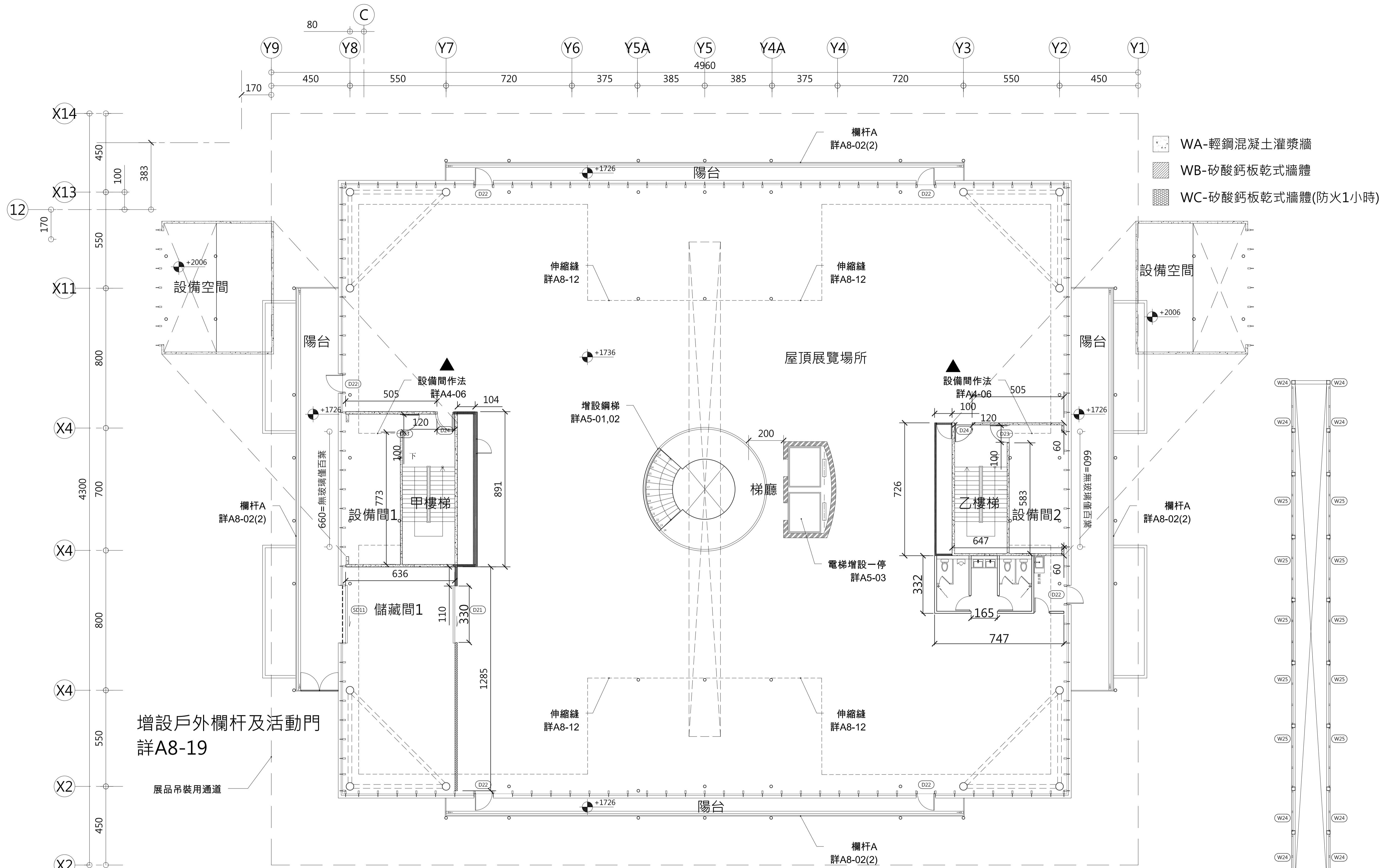
1 屋頂展覽場所平面圖 A1=1/100 UNITS:CM
